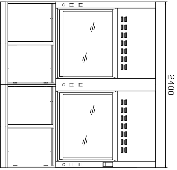
正视图
