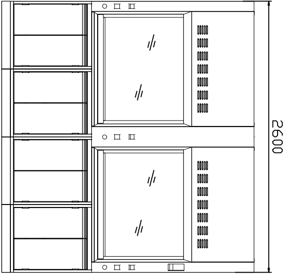
正视图
