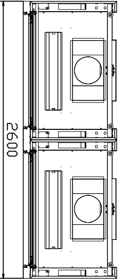
俯视图
