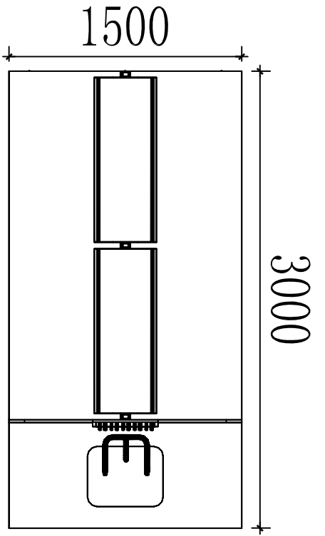
平面图 (316室)
