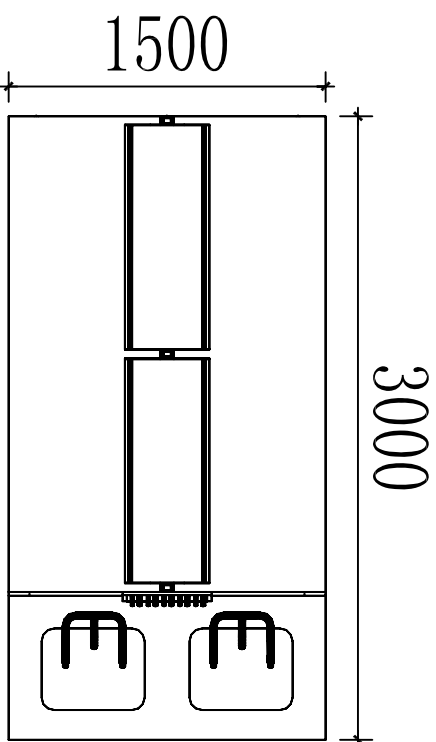
平面图 (512型)
